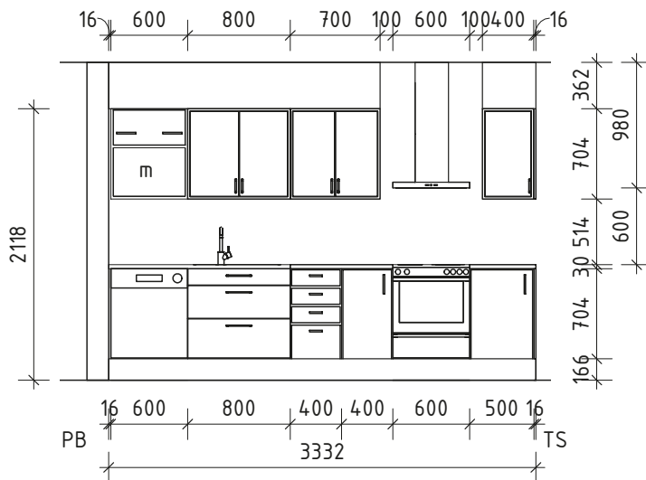
KÖK - K1b ELEVATION A
