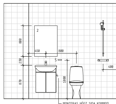
WC/D - TYP 1 - VY 3
