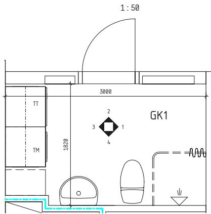
WC/D - TYP 5
