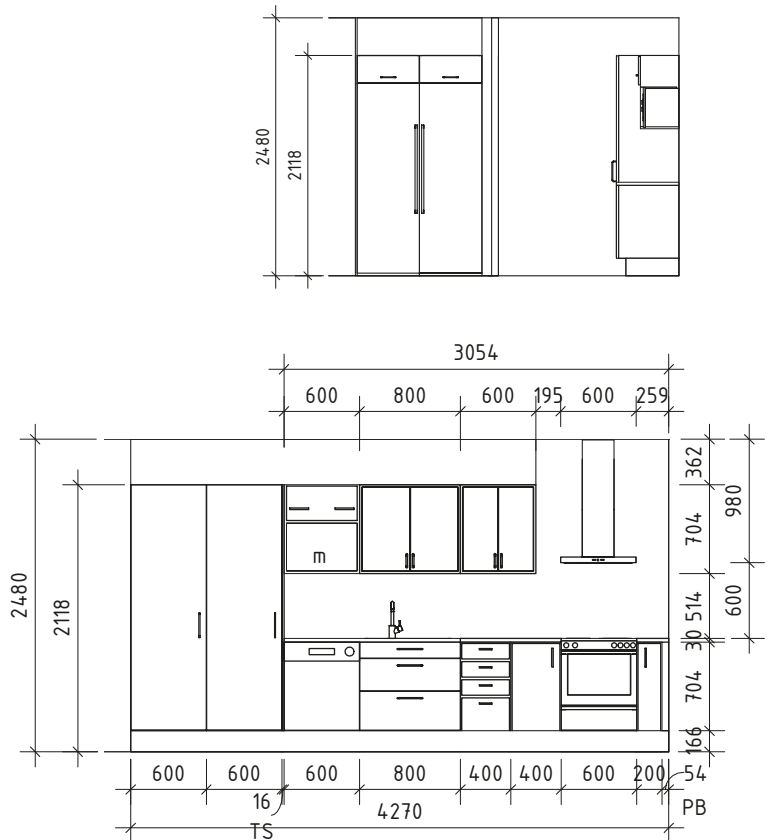
KÖK - K3 ELEVATION B
