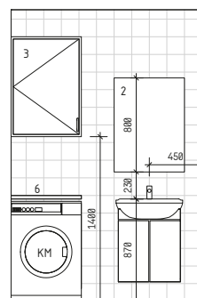
WC/D - TYP 2 - VY 3
